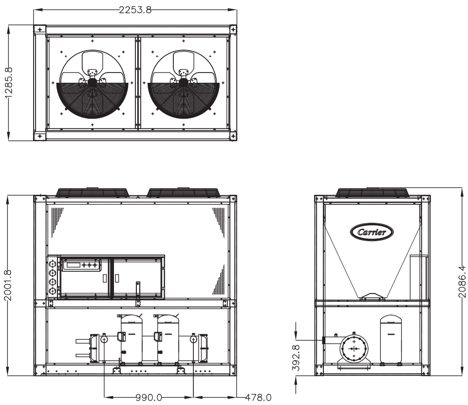
Model : 30GSU018
