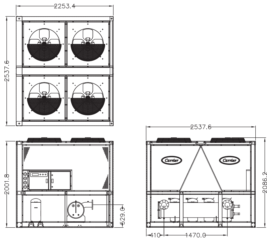
Model : 30GSU048
